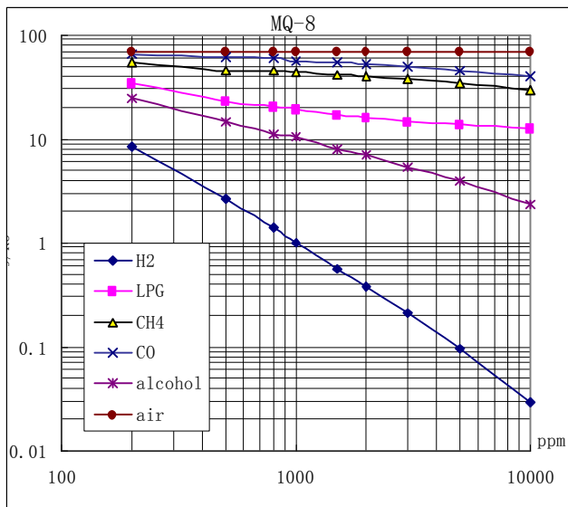
图3 MQ-8型气敏元件的灵敏度特性
